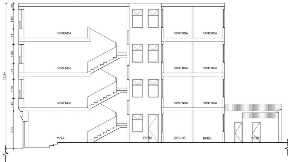
Corte longitudinal
